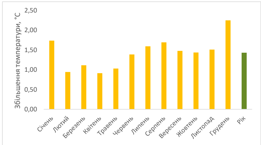
Прогноз змін середніх місячних температур повітря у 2031-2050 рр. порівняно з 1991-2010 рр., °C
