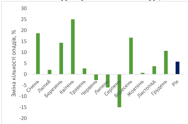
Прогноз змін середніх місячних та річних сум опадів у 2031-2050 рр. порівняно з 1991-2010 рр., %
